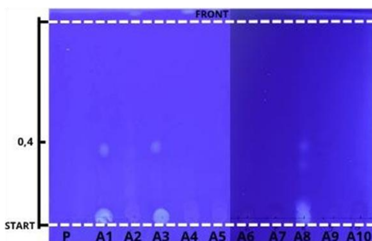
Figura 4: Cromatograma visualizado sob luz UV 364nm . P: Padrão de Epicatequina. Fase móvel: Acetato de Etila, Ácido Fórmico e Água (9:0,5:0,5).
