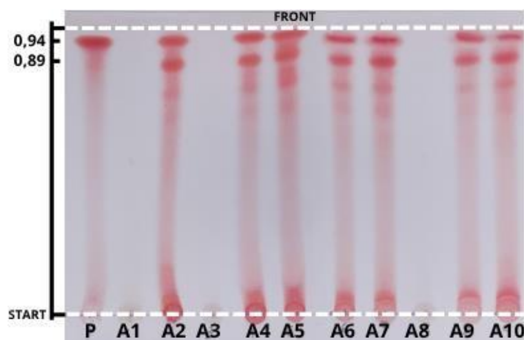
Figura 3: Cromatograma revelado com Vanilina sulfúrica SR. P: Padrão de Epicatequina. Fase móvel: Acetato de Etila, Ácido Fórmico e Água (9:0,5:0,5).
